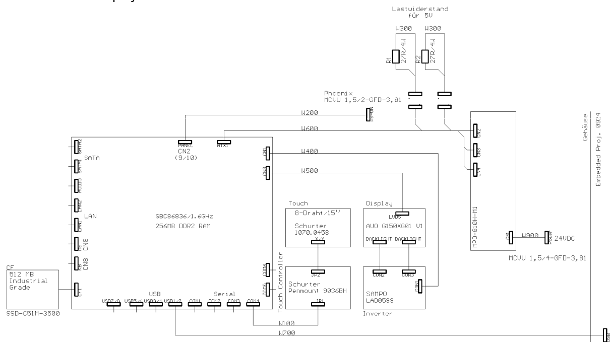
Abbildung 1: Blockschaltbild
