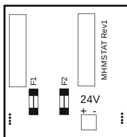
PCB MHM STAT Rev1 90-0-0-9019-0
