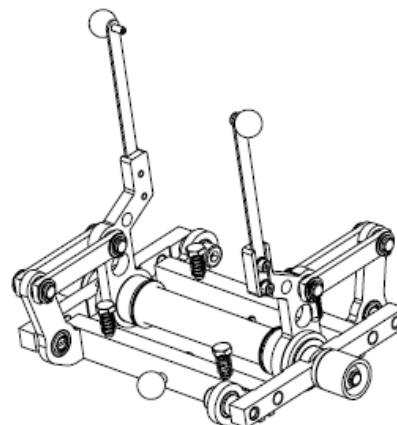
axis for tilty bar Hauptrohr Kippvorrichtung 01-1-6-0004-0
